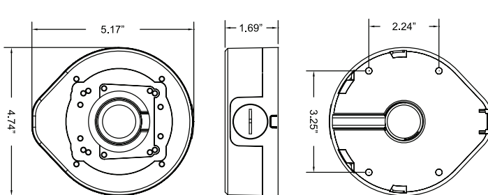
VT-TJB04 Dimensions
