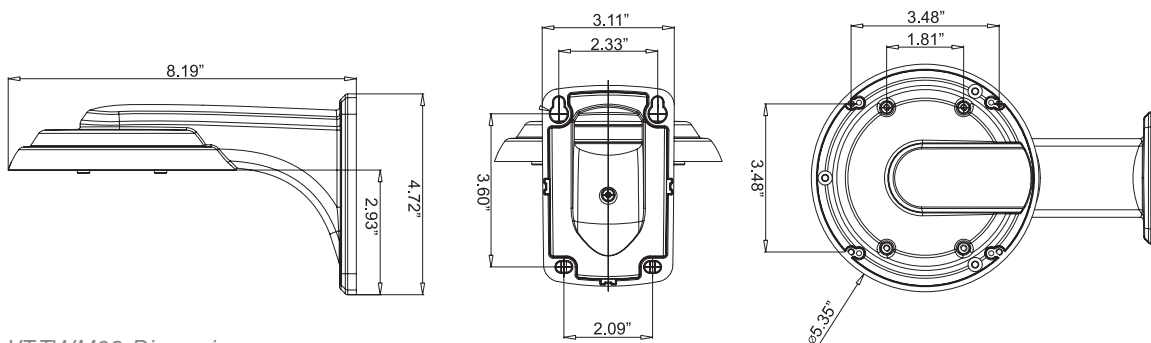
VT-TWM03 Dimensions
