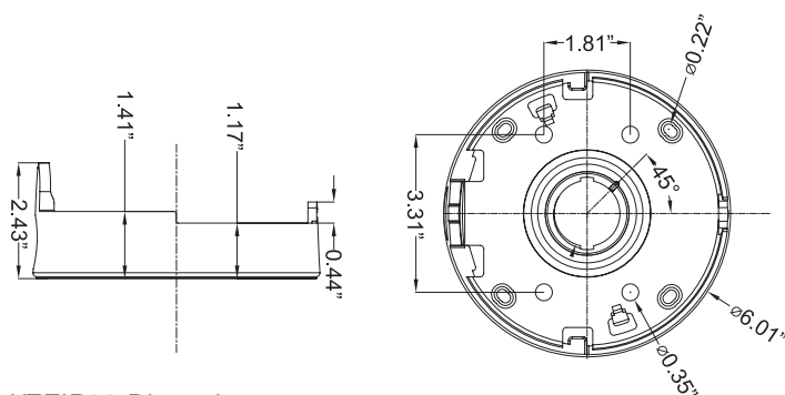
VT-TJB02 Dimensions
