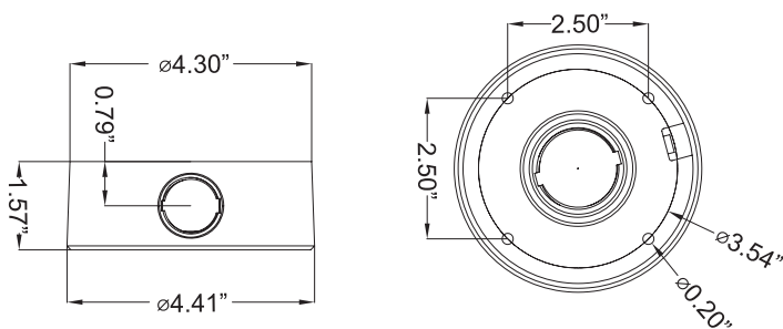
VT-TJB03 Dimensions
