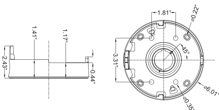
VT-TJB02 Dimensions
