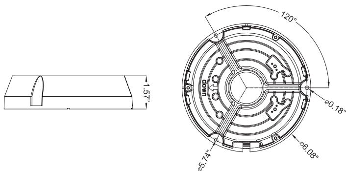
VT-TJB01 Dimensions
