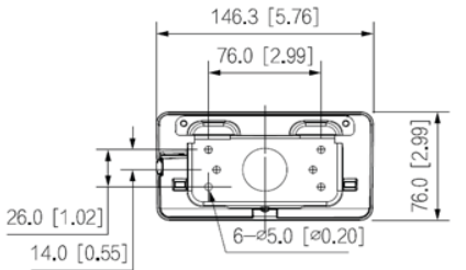
Back View (mm [in.])
